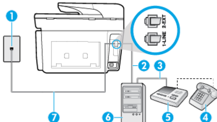
Afbeelding 5-13 Achteraanzicht van de printer
